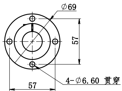
底座安装尺寸
